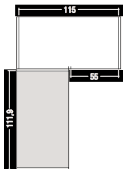
articolo 120 angolo a 90° in TANGANIK A 1 ante battente DX o SX. TANGANIK A 90° corner 1 DX or SX hinged door. cm. h. 256
